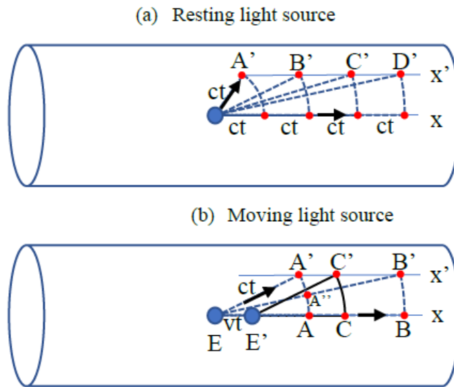
Figure A1. Longitude density of photons
